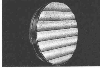
Automatische Verschlussklappe mit austauschbaren Kunststoff- lamellen, langjährige Haltbarkeit, rund u. viereckig lieferbar in 300/350/400/500 mm ø
