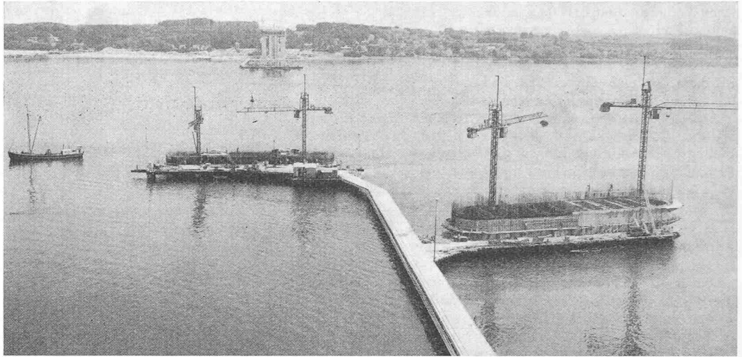
Bild 8. Der Fünen-Pfeiler (rechts) bei seinem Zwischenhalt auf der Reise an den plangemässen Standort (Blick vor der Westrampe nach Osten in Brückenlängsrichtung)
