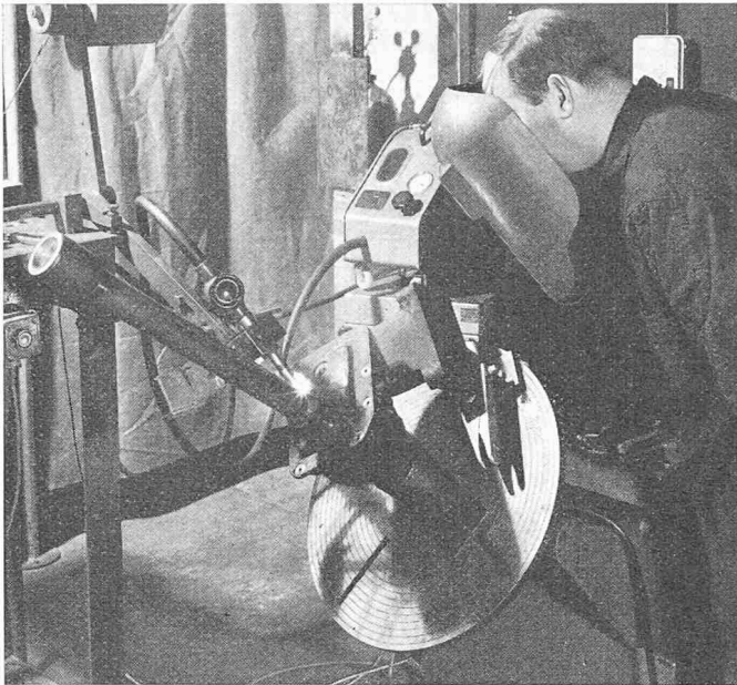
Bild 8. Automatisches Schweißen eines Stahl-Führungsrohres an einem Lenkgehäuse aus Gusseisen mit Kugelgraphit. Werkbild Burmann & Sons Ltd., Birmingham
