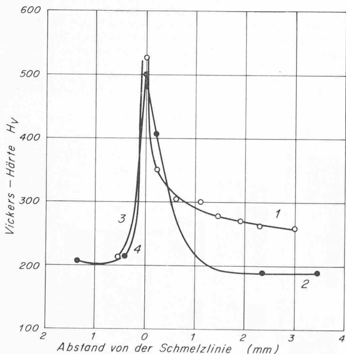
Bild 1. Verlauf der Härte in Funktion des Abstandes von der Schmelzlinie bei einer Schweissnaht an Gusseisen mit Kugelgraphit. Ohne nachträgliche Wärmebehandlung
