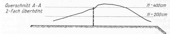
Bild 3. Triebsschneeeablagerungen am 14. April 1967 im Bereich der Triebsschneewände OeAM (H = 400 cm) auf Fachswang, Lawinenverbauung Tanngrindel, Brienz. Die Triebsschneewände stehen ungefähr in der Hangfall-Linie und mehr oder weniger senkrecht zur Hauptwindrichtung. Die mittlere Hangneigung im Bereich der Triebsschneewände beträgt 29°. S = Schneebücken mit Füllungsgrad min. 65 %
