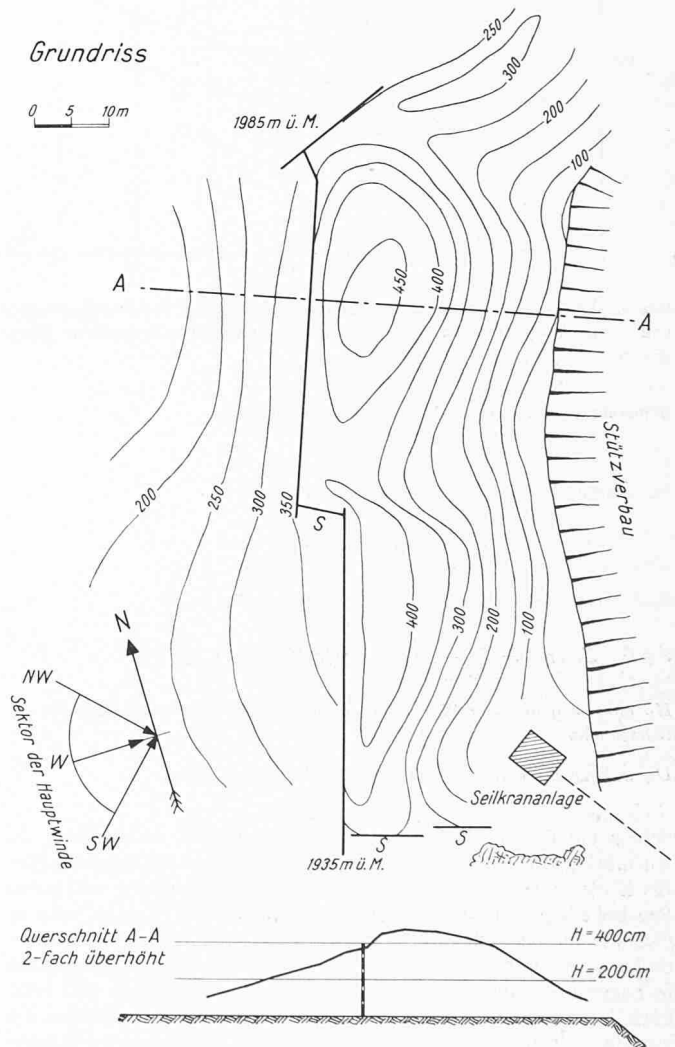
Bild 3. Triebsschneeeablagerungen am 14. April 1967 im Bereich der Triebsschneewände OeAM (H = 400 cm) auf Fachswang, Lawinenverbauung Tanngrindel, Brienz. Die Triebsschneewände stehen ungefähr in der Hangfall-Linie und mehr oder weniger senkrecht zur Hauptwindrichtung. Die mittlere Hangneigung im Bereich der Triebsschneewände beträgt 29°. S = Schneebücken mit Füllungsgrad min. 65 %
