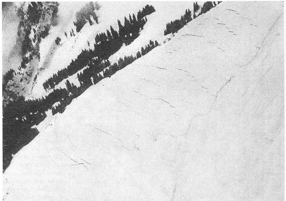
Bild 2. Lawinenniedergang vom 21.3.67 östlich der stark eingeschnittenen Lawinenverbauung Tanngrindel/Brienz. Trotz des offenen Verbaungrandes breitete sich in diesem Fall das Schneebrett mit einer Breitenentwicklung von 1500 m nicht in die Stützverbauung hinein aus. Die seitlichen Anrisslinien fallen mit dem Verbaungrand zusammen; die stabilisierende Wirkung der Stützverbauung auf die Schneedecke ist eindeutig sichtbar. Aufnahme 21.3.67 von W. Schwarz
