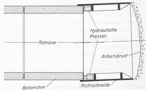
Bild 10. Steuerung des vorderen Rohrelementes durch Richtungsänderung des vorderen Stahlschildes (Richtschnide) mittels hydraulischen Pressen
