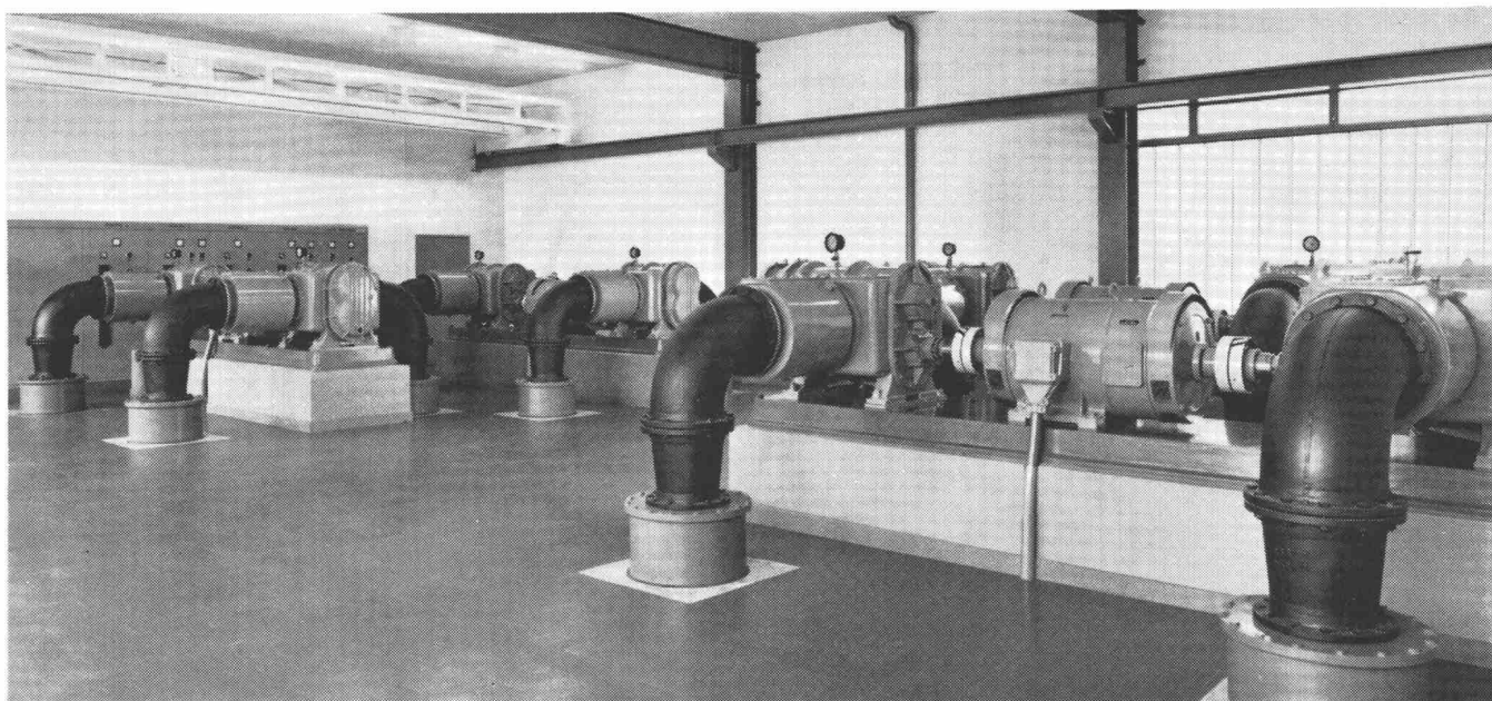
Gebälseanlage, bestehend aus vier Doppelgruppen R 400-400 mit einer totalen Fördermenge von 60 000 m 3 /h, für den Betrieb der Belebtschlammbecken der Kläranlage Hard in Winterthur
