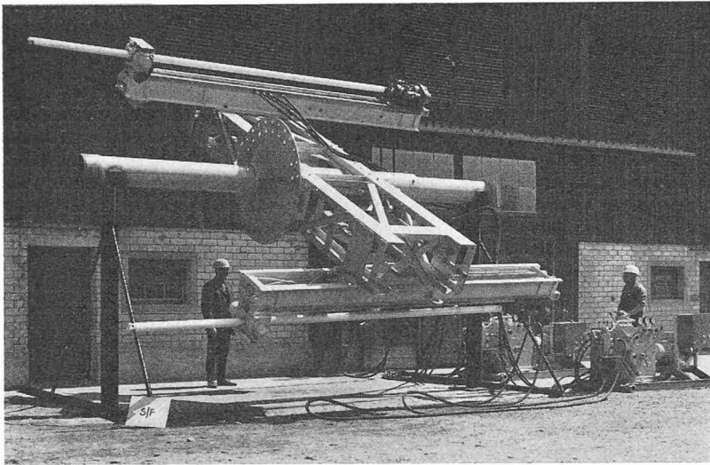
Figure 5. Aménagement de l'Hongrin-Léman, galerie d'adduction Est. Le jumbo rotatif et ses deux perforatrices, pour le forage et la mise en place des congélateurs (document S. I. F. — Photo Germond, Lausanne)
