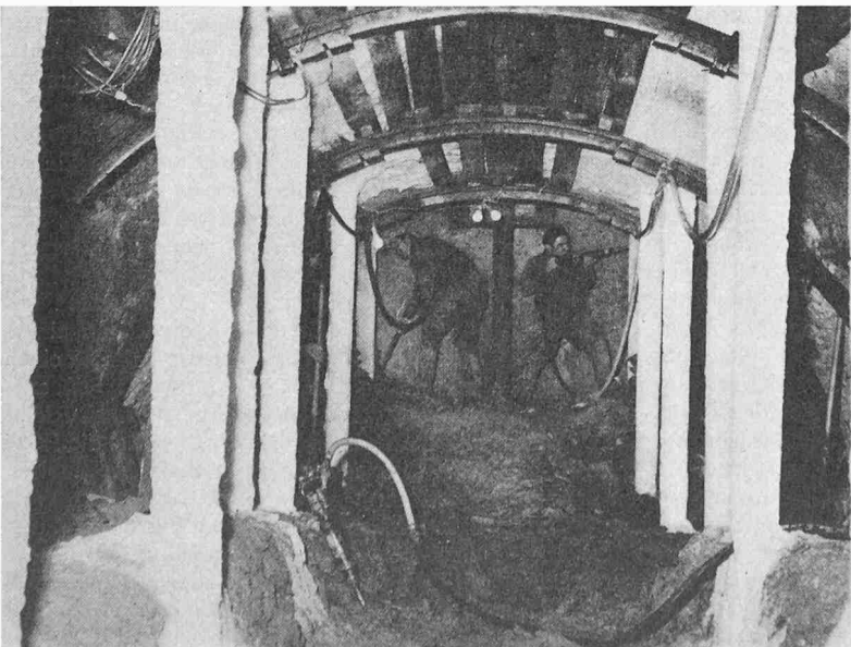
Figure 10. Collecteur souterrain de Watrelos. Creusement de la demi-section supérieure, les congélateurs intérieurs restant en service (document Foramines)
