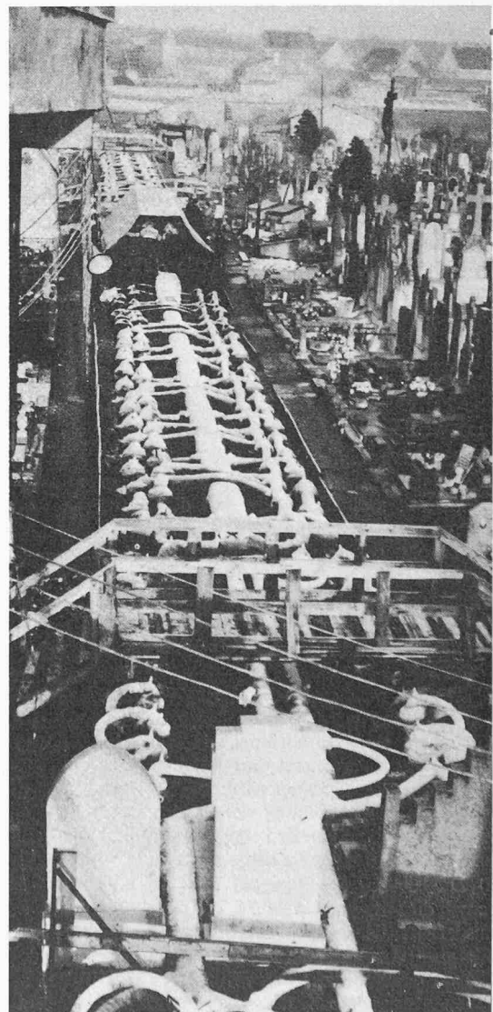
Figure 9 (à droite). Collecteur souterrain de Watrelos, vue générale des équipements de surface pour la congélation (document Foramines)
