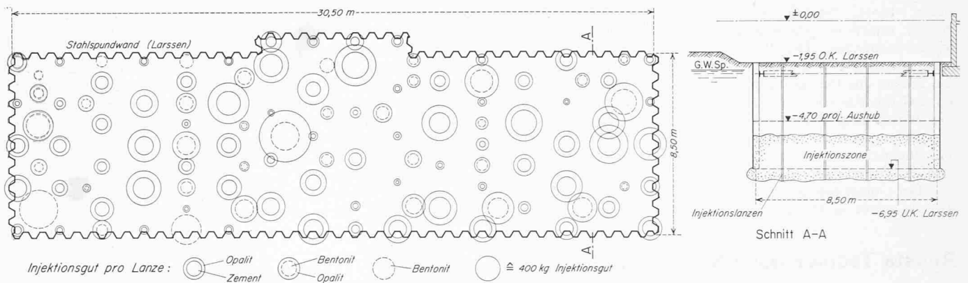
Bild 5. Neubau Wagonfabrik Schlieren, Injektionswanne mit Splundwand (Stump-Bohr-AG). Masstab 1:250
