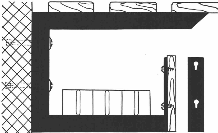
Sitzbank-Konsole mit Konvektorenträger. Frontverschalung auf Bajonettverschluss. Wand- oder Bodenverankerung. Richtpreis Fr. 12.— bis 15.— einbrenngründert.
