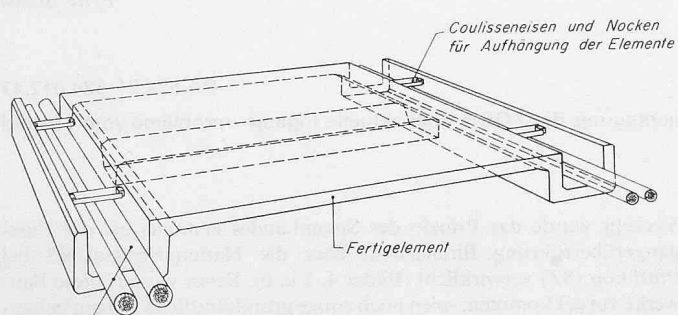
Spannkabel
