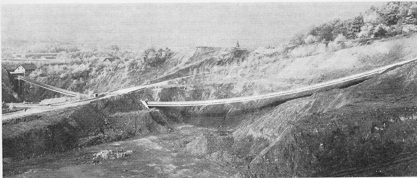
Bild 2. Transportbandbrücke der Cementfabrik Holderbank-Wildegg. Da hier ein grosser Durchhang zulässig war, konnte das 216,4 m lange, auch im Stollen (Bildmitte) freihängende Spannband mit geringem Spannstahlaufwand wirtschaftlich gebaut werden
