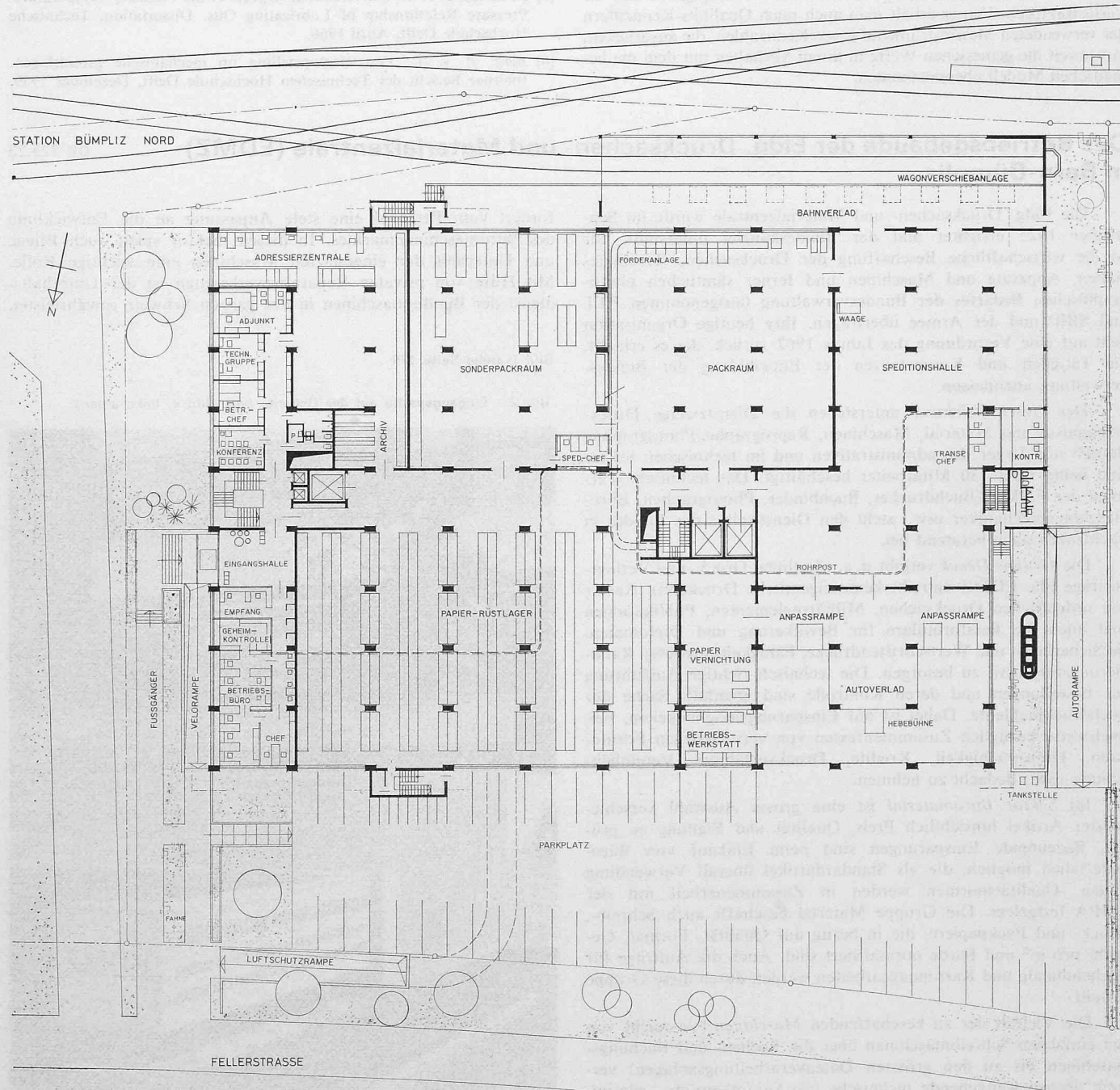
Bild 4. Erdgeschoss 1:600 mit Haupteingang, Verwaltungs- und Betriebsbüros, Adressierzentrale, Pack- und Speditionsräumen, Papier-Rüstkammer sowie Bahn- und Autoverlad
