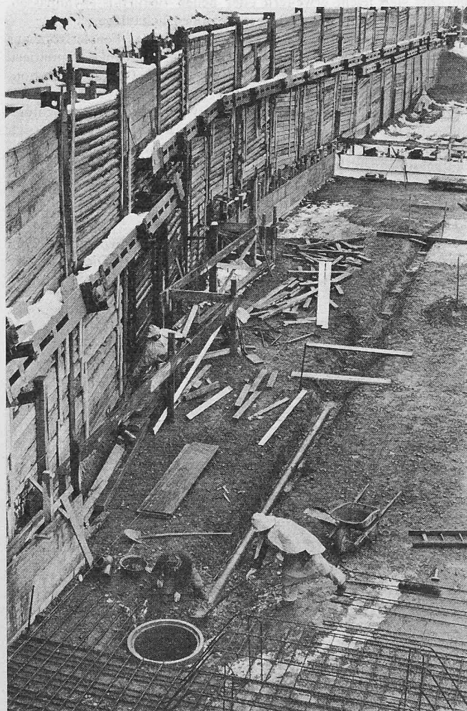
Bild 12. Die Südseite der Baugrube mit Rühlwand
