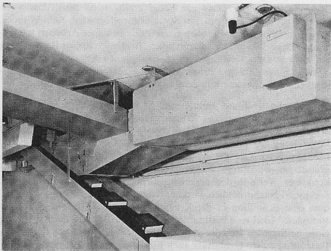
Bild 40. Übergangsstelle eines horizontalen Förderbandes (oben links) zum Steigband; rechts oben das zugehörige Antriebsaggregat; unten links das Steigband des unteren Geschosses
