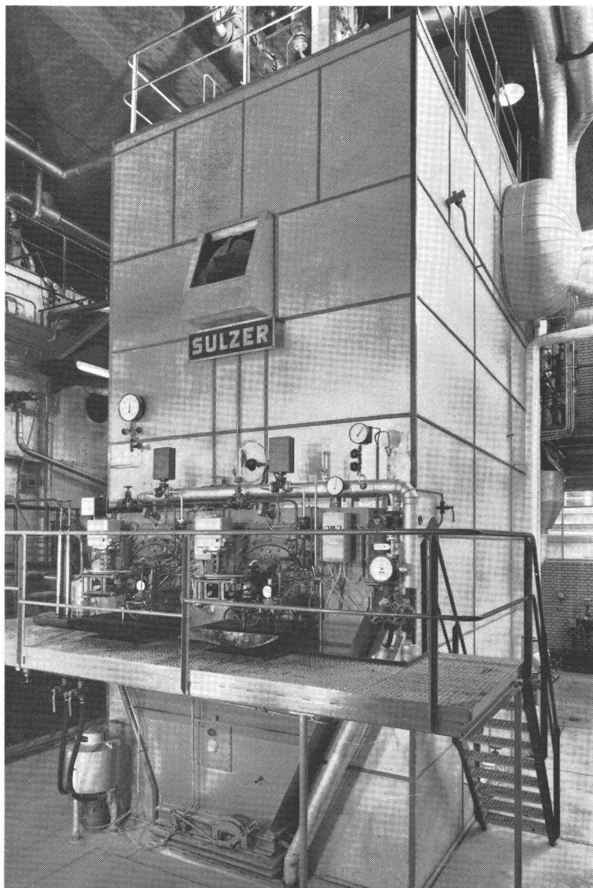
Sulzer-Hochleistungs-Strahlungskessel mit Überdruckfeuerung und Bedienungs- und Bedienungspodest für 2 Sulzer-Ölbrenner von je 800 kg Öl/h in einer Kartonfabrik. Kesseldaten: 16 bis 20 t/h, 41 atü, 425 °C.
