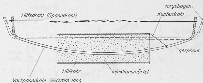
Bild 10. Biegelprobe zur Bestimmung der Umschlagbiegezahl, mit der Anordnung von Hüllrohr, Injektionsmörtel und leitender Verbindung. Reproduktion der Verhältnisse am Objekt
