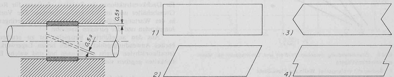
Bild 7. Bewährte Einbauverhältnisse und Foliendicke für Schlitzringlager aus PTFE. Links Einbauverhältnisse, s Foliendicke. 1 bis 4 typische Querschnitte
