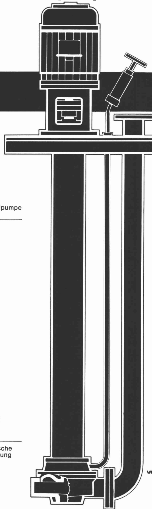
2 HÄNY-Normschacht
