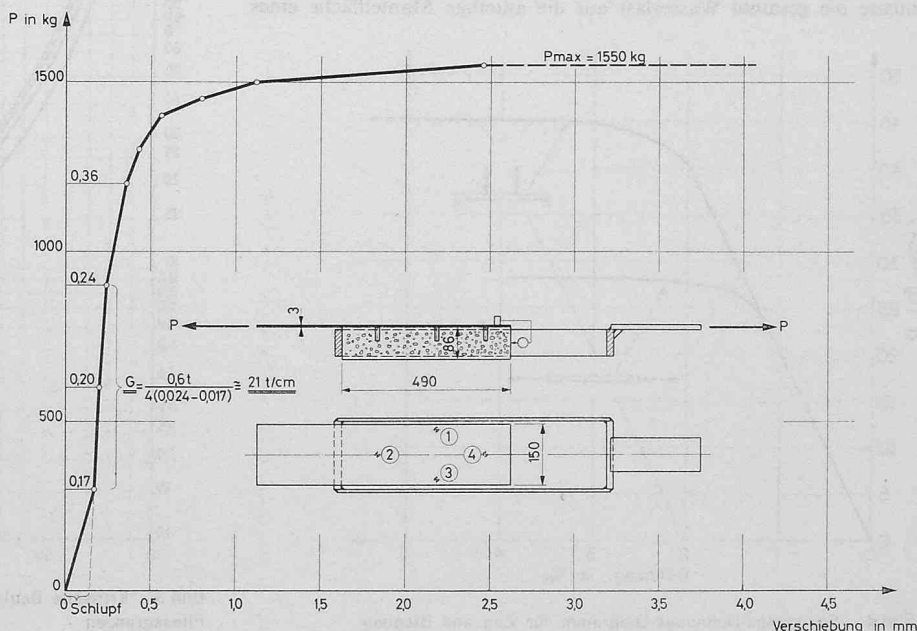
Bild 10. Belastungs-Verschiebungs-Diagramm der Dübel
