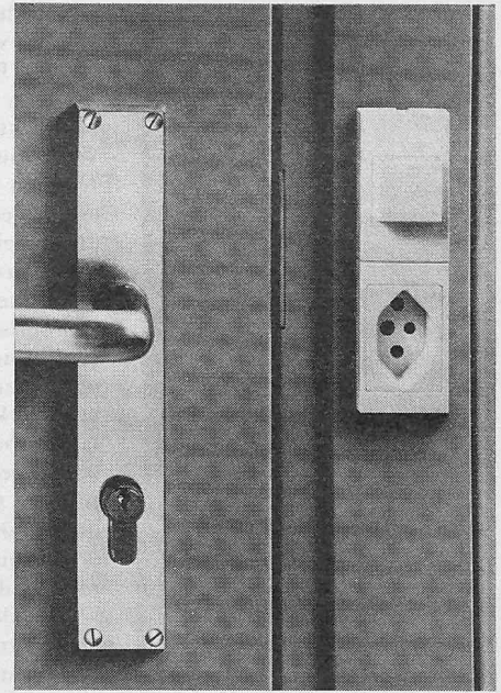
Bild 2. Druckschalter und Steckdose in der Türzarge
