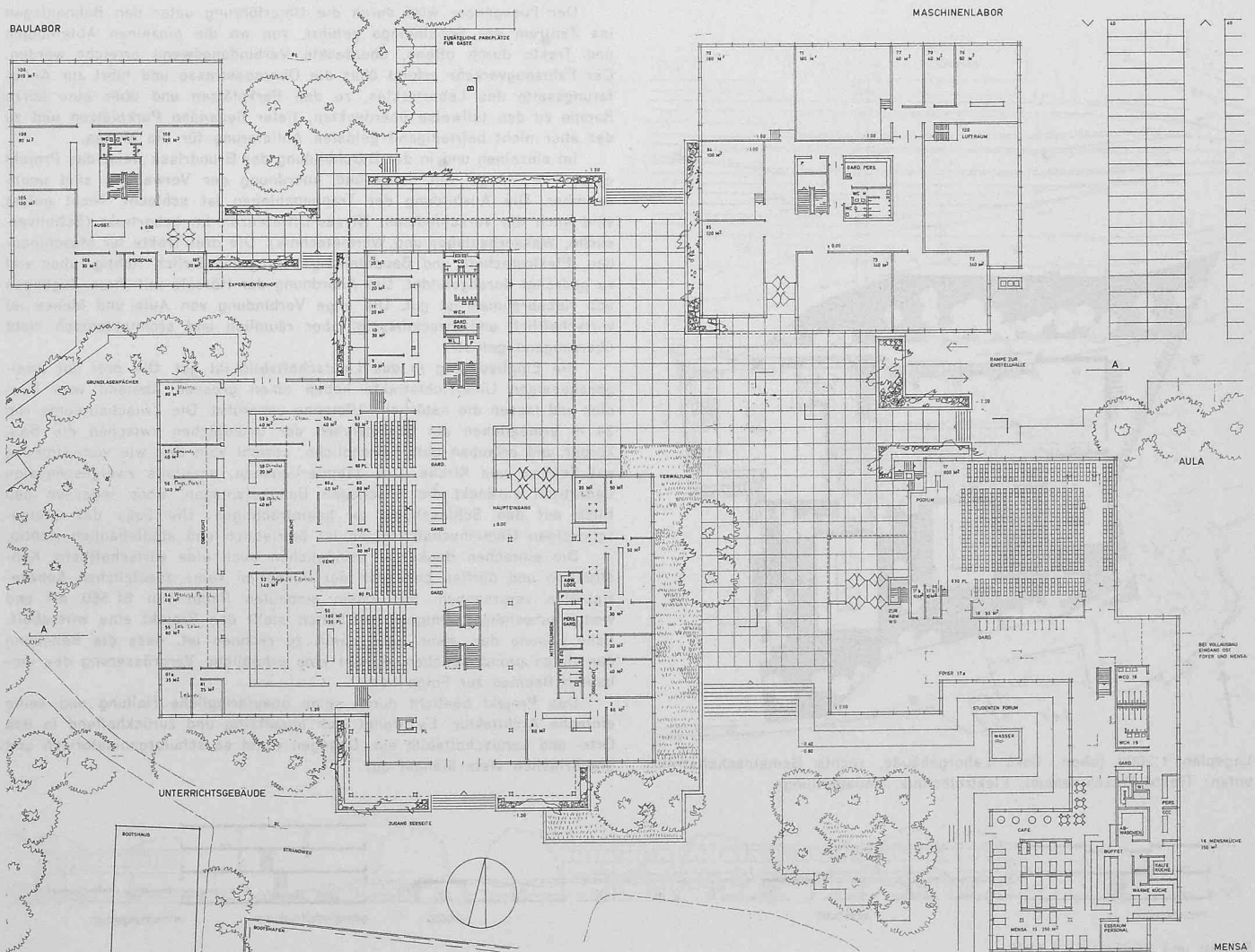
Erdgeschoss (Gesamtanlage) 1:1000
