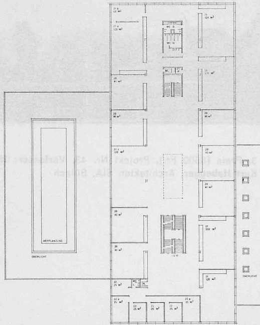
Unterrichtsgebäude, 1. Obergeschoss 1:1000
