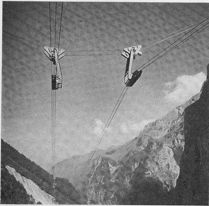
Bild 3. Einzelheit der Hängestütze Sandalp
