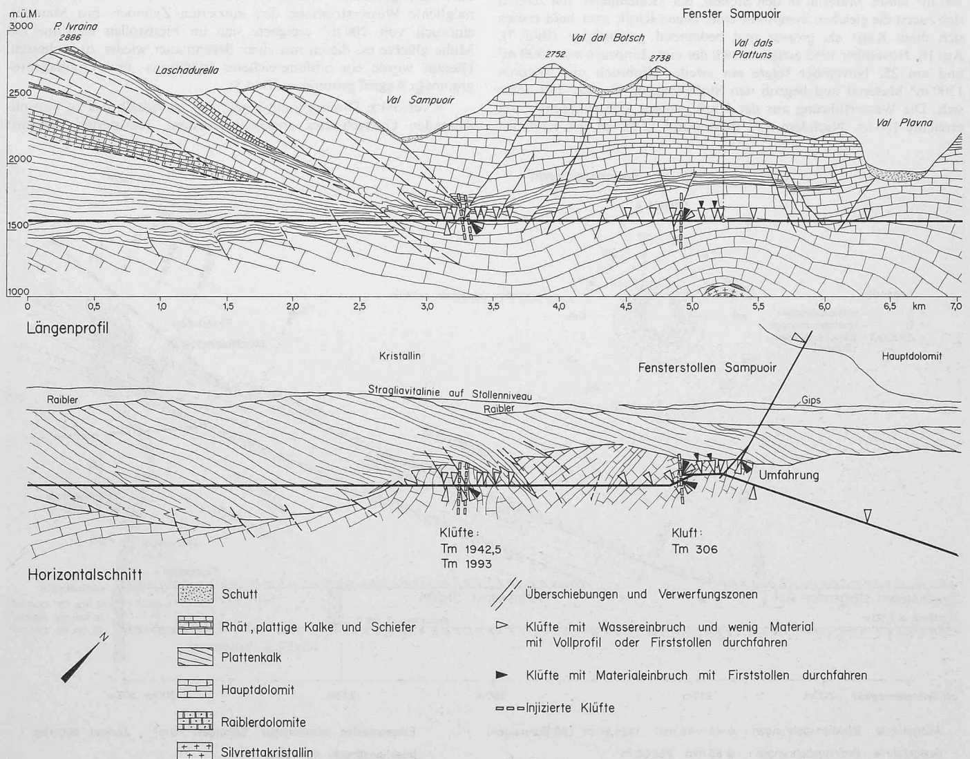
Bilder 5 und 6. Druckstollen Sampaioir. Geologische Schnitte 1:40 000 von E. Weber, Geologe, Maienfeld
