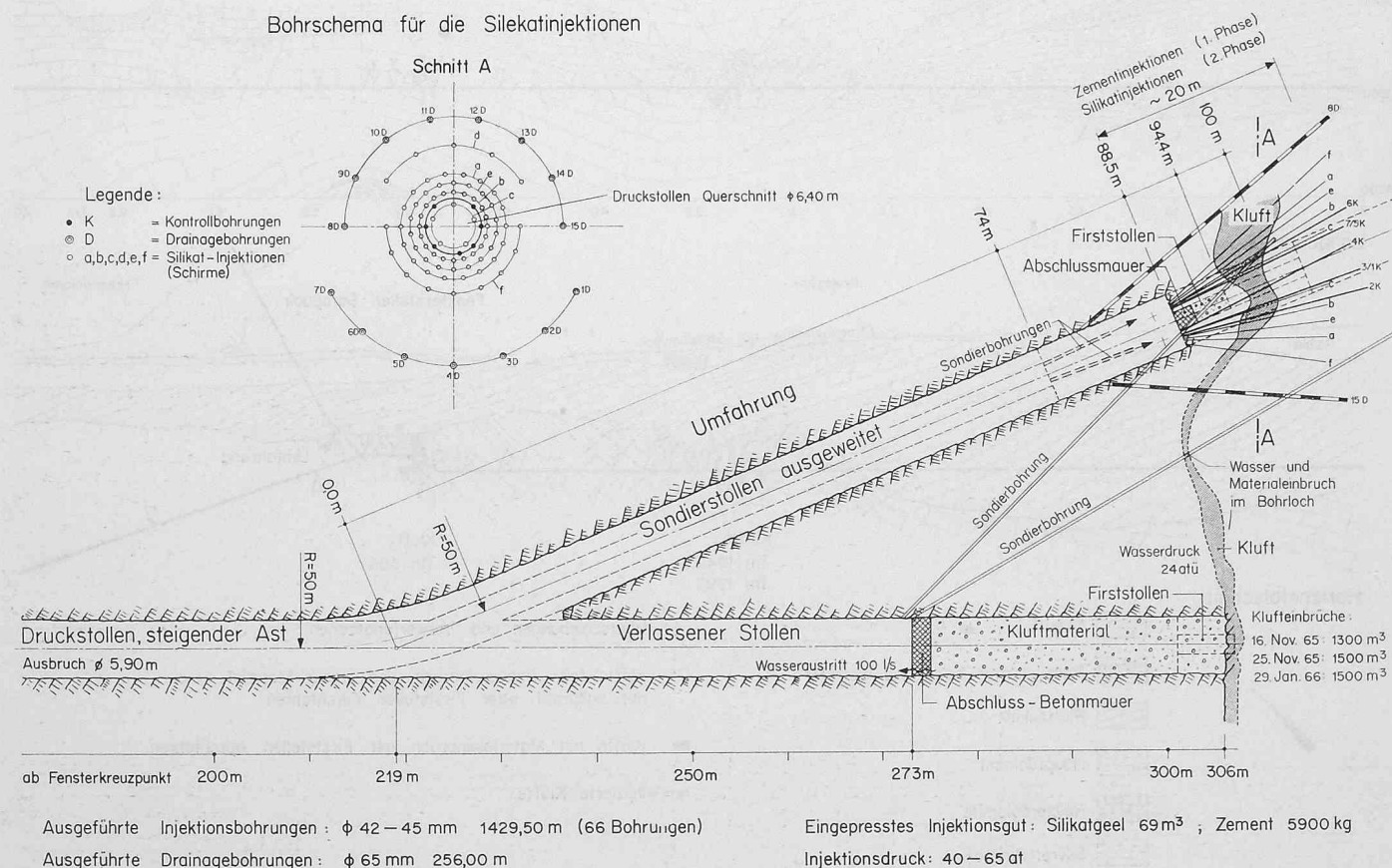
Bild 7. Druckstollen Sampuoir. Einbruchstelle Kluft Stollenmeter 306 mit Umfahrung und Bohrschema für die Silikatinjektionen. Massstab 1:600
