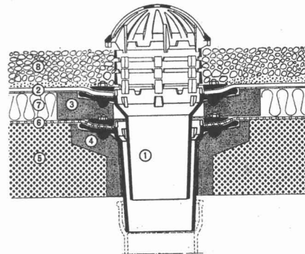
Zweiteiliger Standard-Dachablauf im Kiesschüttdach
