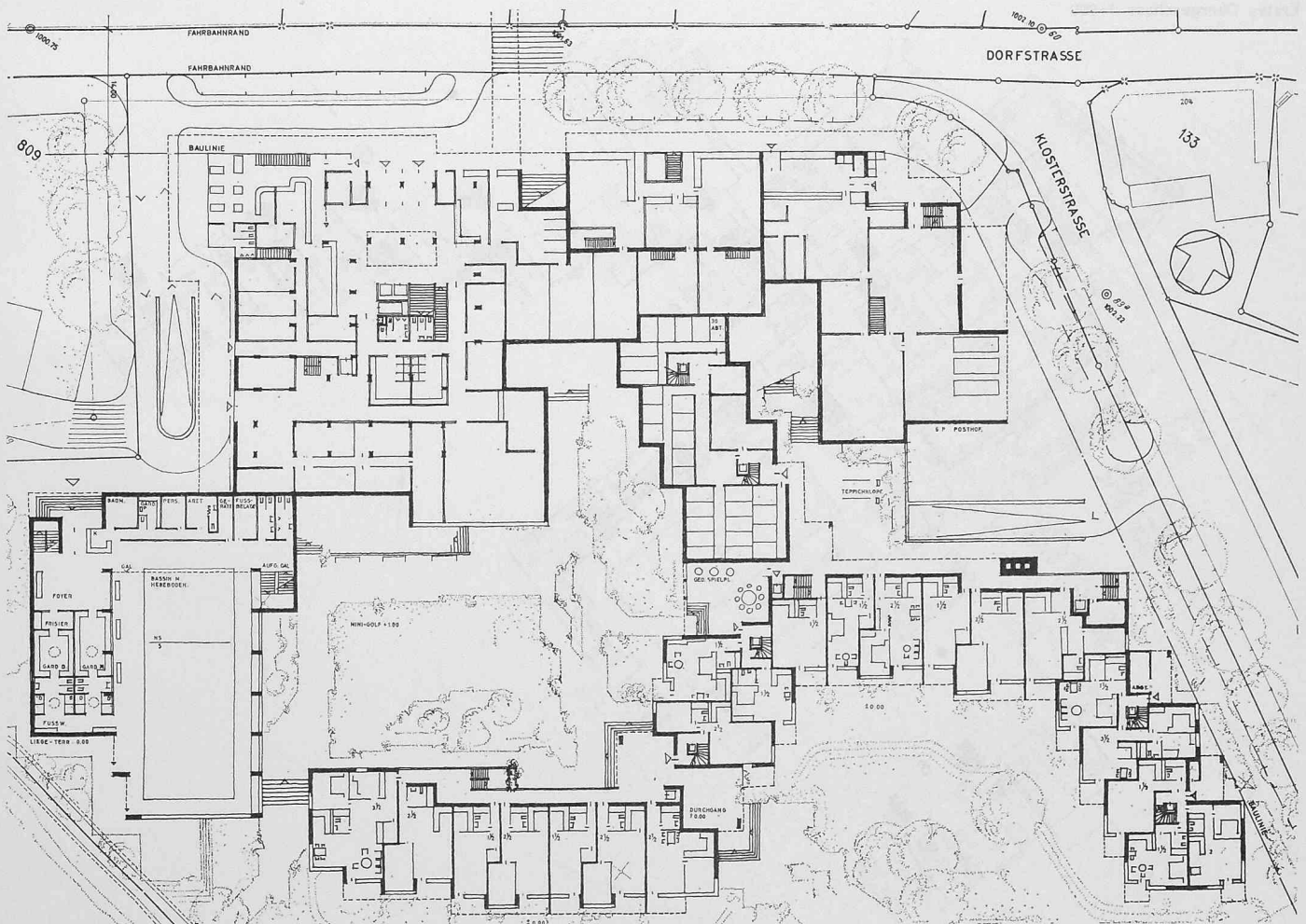
Erdgeschoss 1:800
