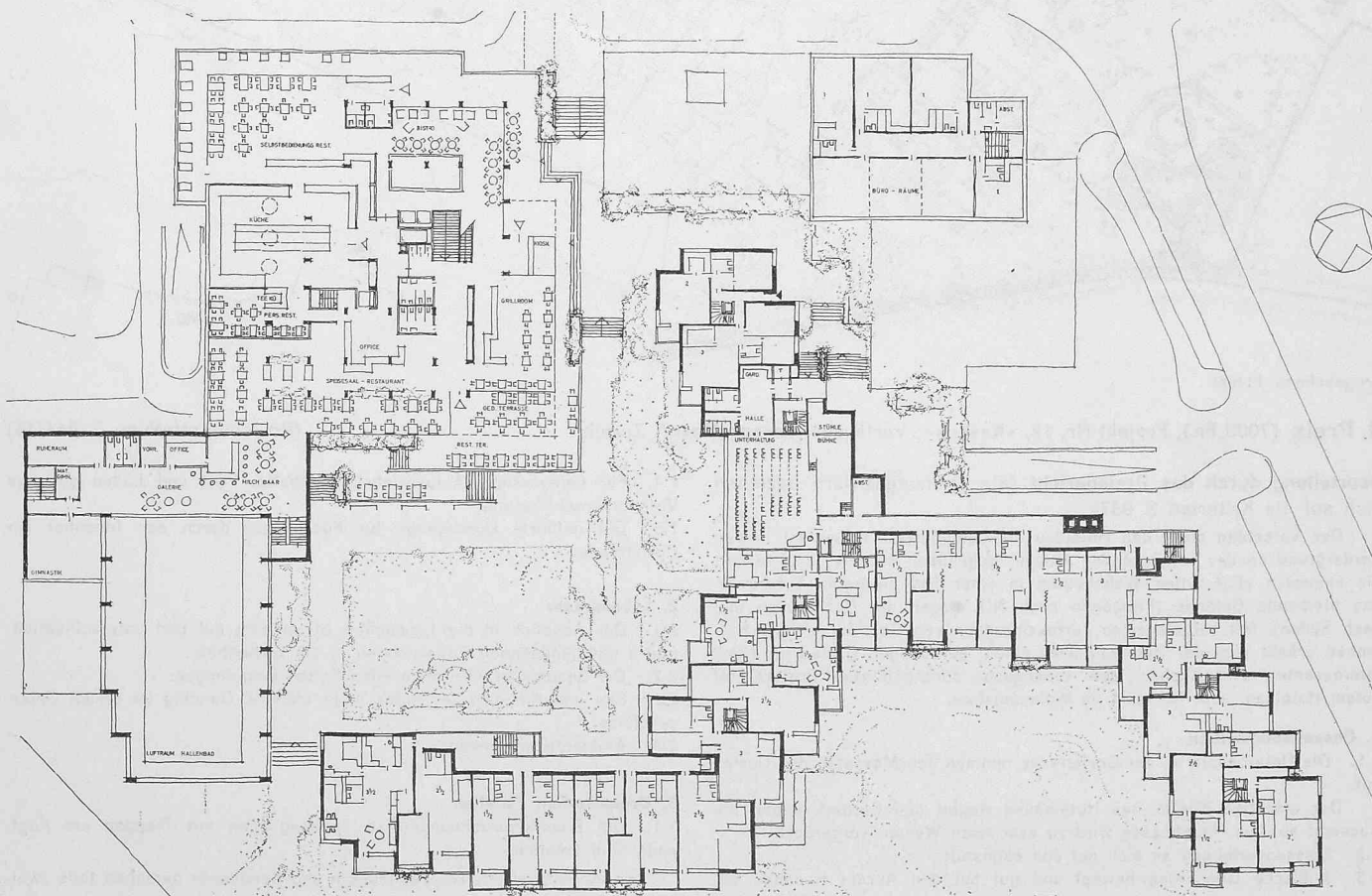
Erstes Obergeschoss 1:800
