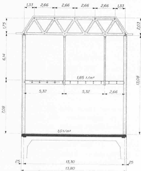
Bild 2. Querschnitt 1:300 durch das aufgestockte Gebäude
