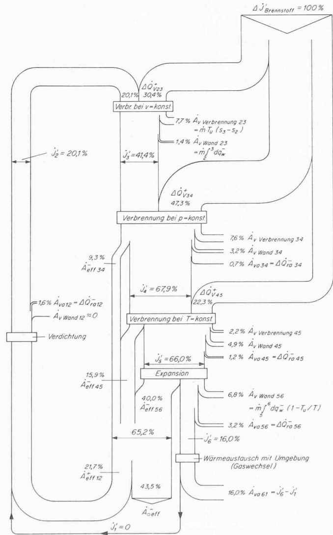
Bild 18. Das Koenergie-Diagramm für den geschlossenen Dieselprozess als Leistungs-Diagramm mit dem sekundlichen Massenstrom \dot{m} = \dot{m} z v
