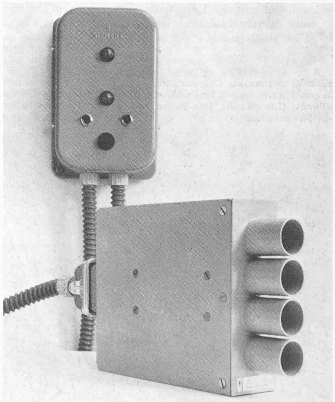
Bild 7. Siemens-Laserlicht-Empfangseinrichtung (LGE)
