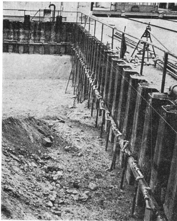
Grundwasser-Absenkung mittels Vakuum-Rohrbrunnenanlage (Wellpoint)
