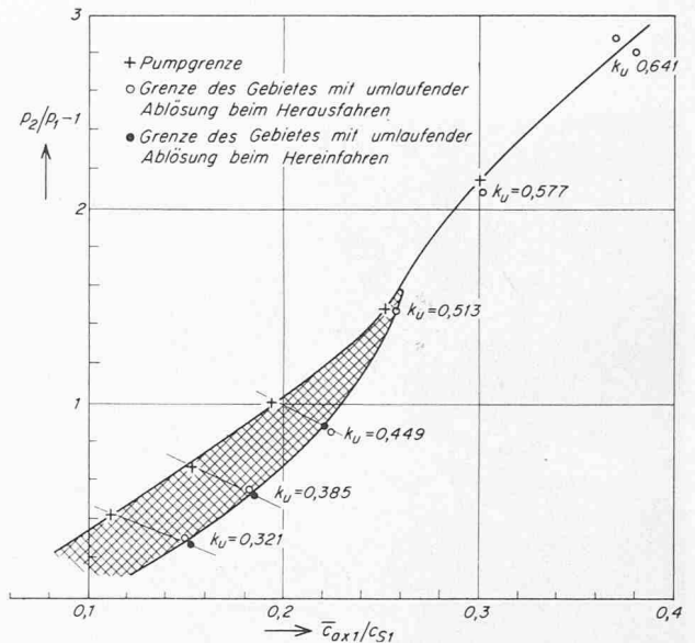
Bild 5. Druckerzeugung p_2/p_1-1 und Gebiet der umlaufenden Ablösung in Abhängigkeit von der relativen Schluckziffer \bar{c}_{ax1}/c_{S1} für verschiedene Drehzahlkoeffizienten k_u . Reynoldszahl Re = 0,5 bis 0,7 \cdot 10^6
