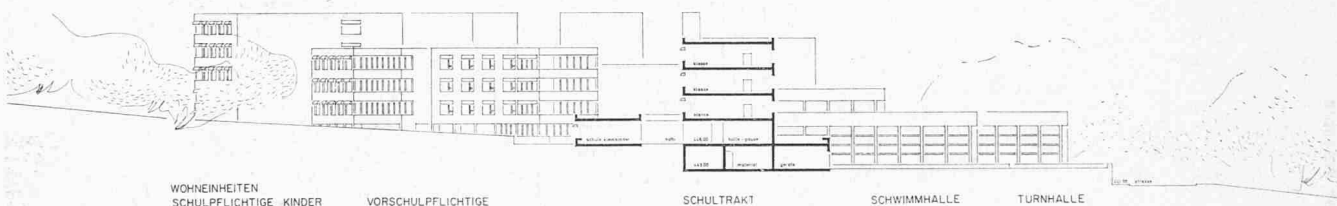
Schnitt 1:900 mit Ostansicht
