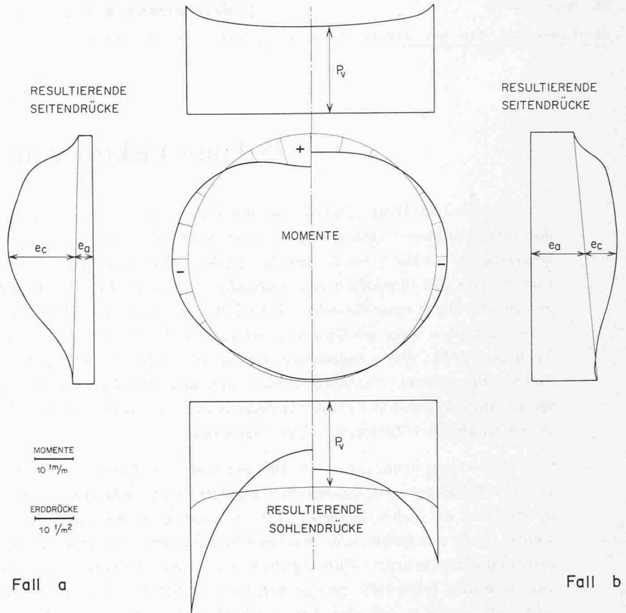
Bild 4. Momente, Seiten- und Sohlendrucke
