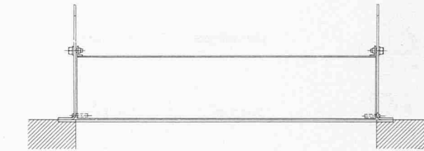
Bild 8. Einstellbare Abluftklappe für den Einbau in die Tunnel-zwischendecke (Konstruktion Luwa AG)
