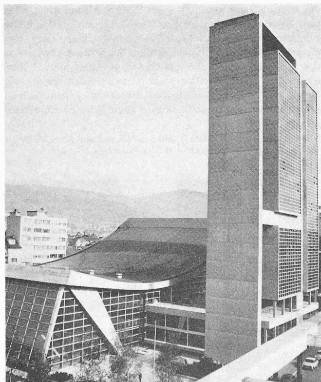
Der Komplex Hallenschwimmbad/Kongresshaus mit Hängedach und Schrägfassade der grossen Schwimmhalle sowie das Bürohochhaus von Südwesten (s. SBZ 1967, H. 23, S. 410).
