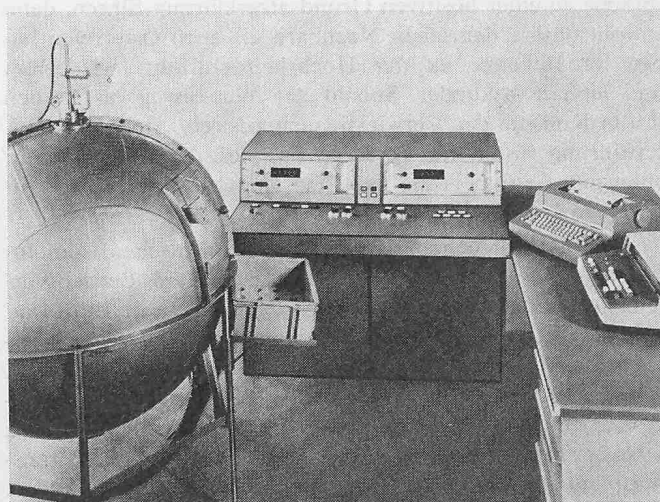
Bild 2. Neuzeitliche, automatische Photometrieranlage in der Fabrik in Winterthur zur Ermittlung von Glühlampen-Kennwerten
