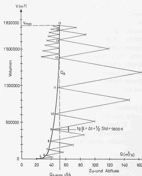
Bild 10. Retentionsrechnung zu Bild 9 im V, Q -Diagramm
