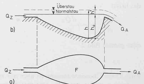
Bild 1. Schematische Darstellung eines Sees in Grundriss a) und Längsschnitt b)
