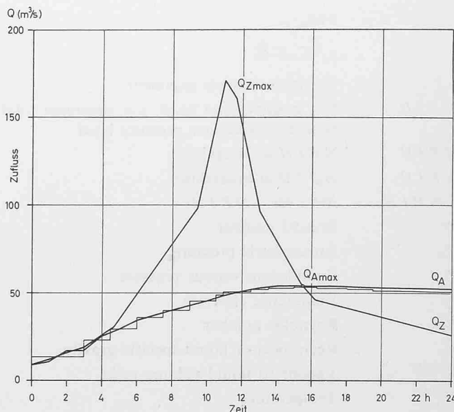
Bild 9. Zu- und Abflussganglinie des Hochwasserretentionsbeckens Orden
