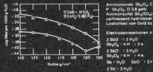
Fig. 14 Löslichkeitskurven und Antimonionen in Schwefelsäure nach Ruetzsch und Angstadt (1)
