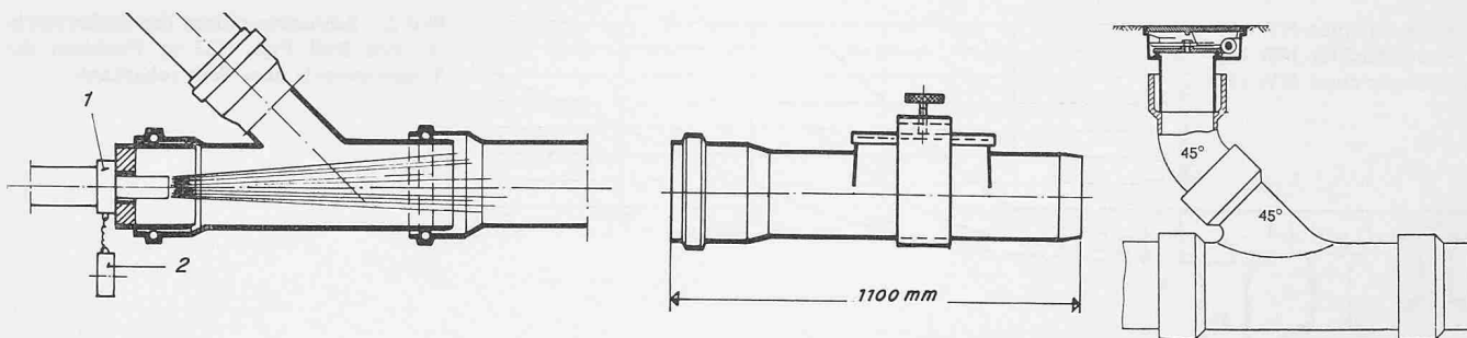
Bild 9. Links: Spülstutzen für die Reinigung der Sammelleitung. 1 Spülschlauch (Feuerwehrschiach), 2 Storz-Kupplungsdeckel; Mitte: Formstück mit Kontroll- und Putzverschluss; rechts: Anordnung eines Reinigungs- und Spülschachtes in der Fahrbahn
