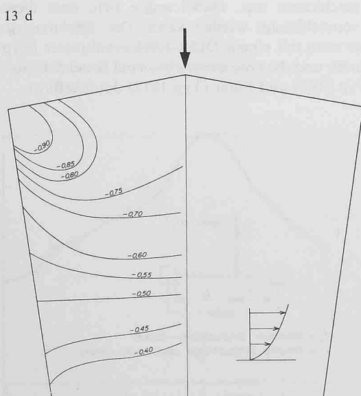
Bild 13. Strömungsbild und stationäre Druckverteilungen (p - p_\infty)/q_{ref} für beide Anströmgeschichten, \alpha = 0^\circ
