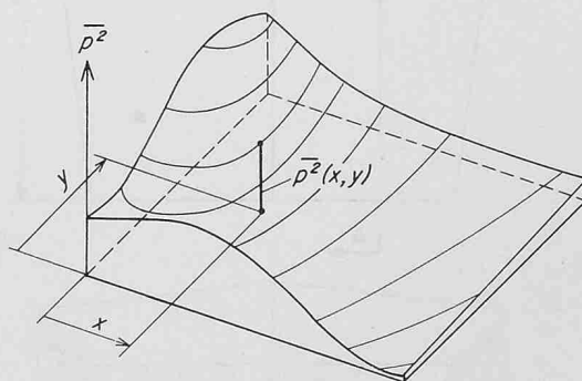
Bild 6. Berechnung der Lastschwankung für eine Fläche mit kontinuierlicher Druckverteilung
