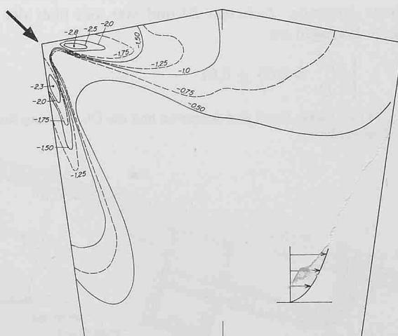
Bild 14. Strömungsbild und stationäre Druckverteilungen (p - p_\infty)/q_{ref} für beide Anströmgeschichten, \alpha = 45^\circ
