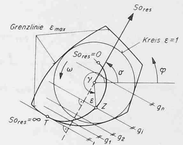
Bild 5.1. Ermittlung der Gumbelkurve für ein segmentiertes Radial-lager
