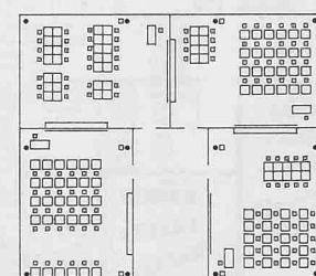
Geschoss E 1:600 (Klassenfrakt 1)
