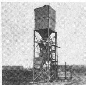
Zwangsmischeranlage
