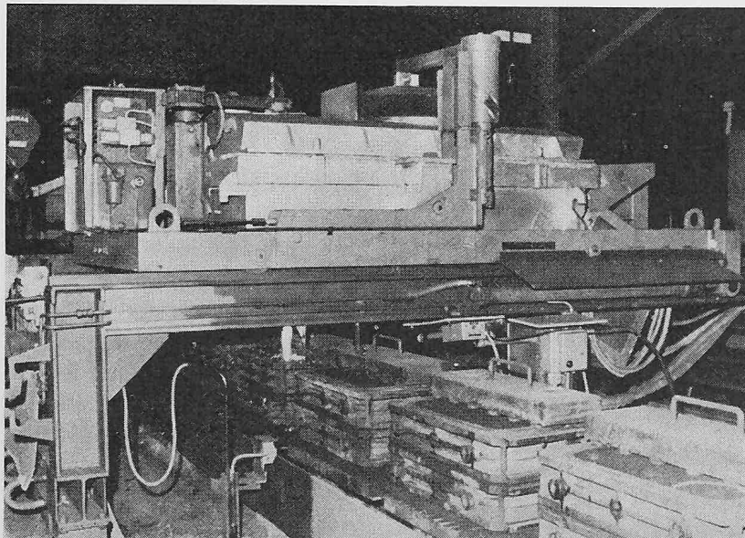
Bild 1. Induktiv beheizte Vergiessereinrichtung zum dosierten Abgiessen von Metallen (Photo Brown Boveri)
