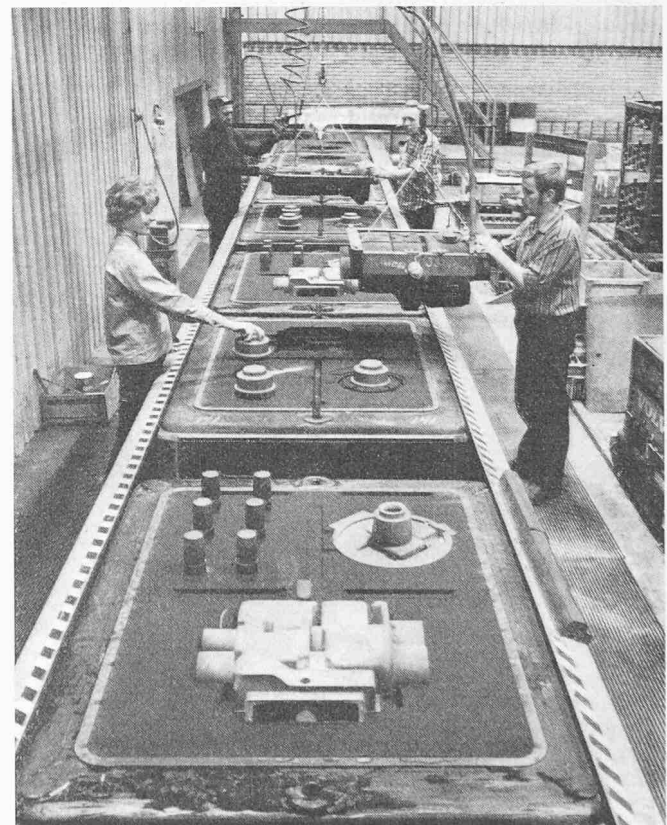
Bild 2. In der Kernmacherei werden die Kerne in die Formen gelegt. Dann werden die Formen automatisch zum Vergiessen transportiert
