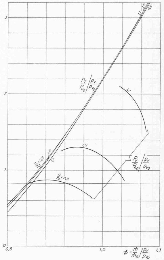
Bild 10. Auf die Nutzleistung P_{n0} = 29,99 kcal/kg und den Eintrittsdruck p_{V0} \approx 9 at (beide Werte bei Normlast) bezogene Leistung der Turbine und des Verdichters
