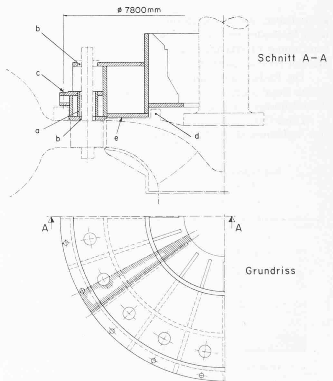
Bild 1. Gehäuseoberteil einer Pumpenturbine für ein hydraulisches Kraftwerk. Die Elementberechnung wird an einem Berechnungsausschnitt (schraffierte Fläche im Grundriss) mit eindeutig bestimm- baren Randbedingungen durchgeführt
