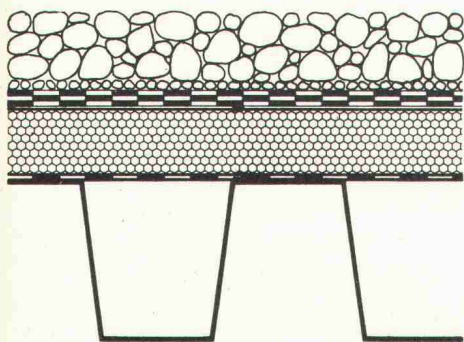
Warmdach Beispiel: Isolierung auf Trapezblechen
