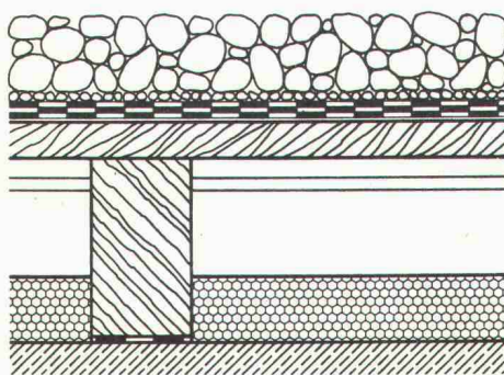
Kaldach Beispiel: Isolierung auf Stahlbetondecke
