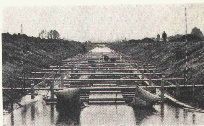
Bild 2. Schwimmende Verlegevorrichtung für die Auskleidung des Kanalprofils mit VSL-Betonmatten
