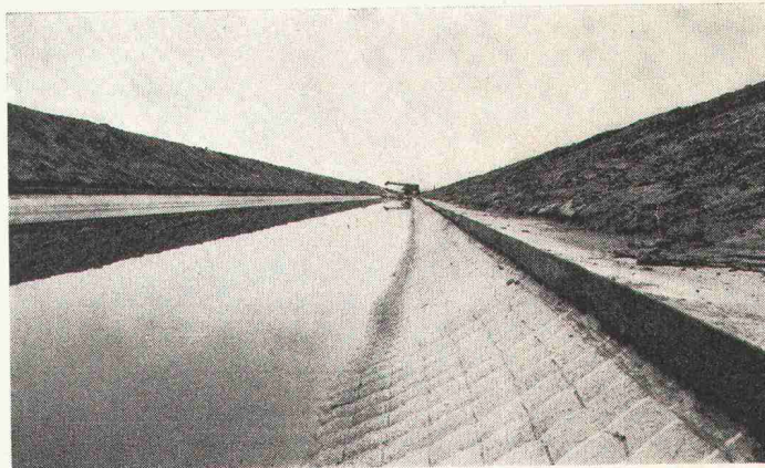
Bild 3. Gesamtansicht der Kanalauskleidung mit VSL-Betonmatten. Die Betonbalken begrenzt die Auskleidung gegenüber dem Terrain
