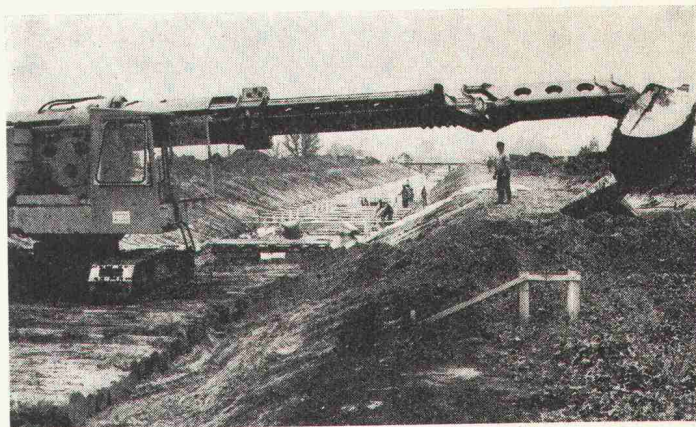
Bild 1. Aushub des Kanalprofils durch Teleskop-Bagger
