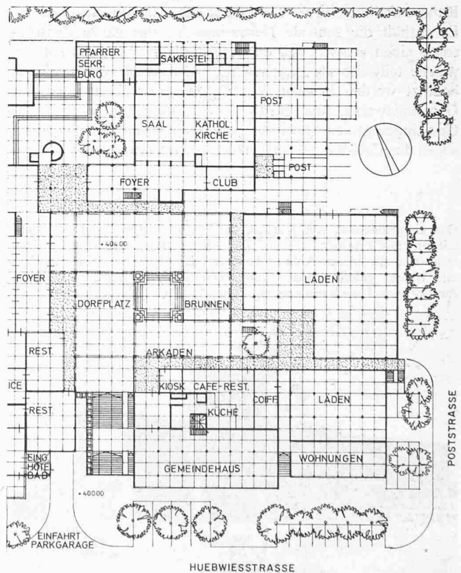
Rechts: Situations-Ausschnitt 1:1200 (Platzgeschoss). Projektierte Ladenstrasse im Zusammenhang mit dem bereits erstellten Gemeindehaus und den im Rohbau befindlichen Gebäuden der katholischen Kirche und der Post
