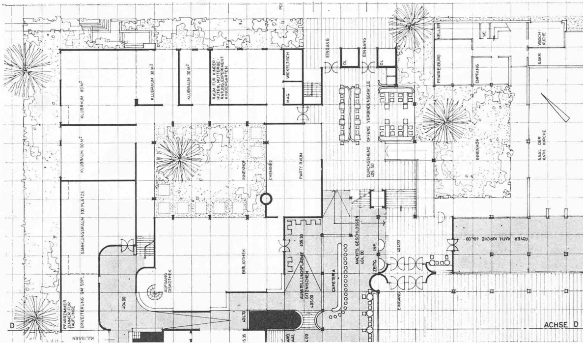
Vorprojekt Freizeitzentrum, Erdgeschoss 1:1000 (Platzgeschoss). Architekten Robert Briner, Herberth Wirth , Zürich. Die reformierte Kirche plant direkt anschließend an den Saalbau der Gemeinde (ab Achse D: Siehe auch Platzgeschoss Hotel/Saal, Bild nächste Seite oben, um 90° gedreht!) nebst einem kleinen Sammlungsraum mit Nebenräumen und Wohnungen ein Freizeitzentrum, welches umfasst: Foyer und Begegnungsraum, Gemeindebibliothek, Partyraum, Kinderhütendienst, Klubraum, Jugendklub, Kegelbahn, Werkräume, Autowerkstatt.
