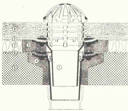
Kiesschüttdach, 2teilig
