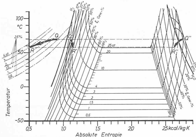
Bild 6. Darstellung der Hilfsgas-Absorption. Die Zustandsänderung des Dampfes ist durch die Linie Q' R', diejenige der Flüssigkeit durch die Linie Q R angegeben. Die Hilfslinien auf der linken Seite entsprechen der isobaren Gegenstromabsorption bei den verschiedenen Drücken, die die Hilfsgas-Absorption durchläuft
