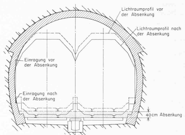
Bild 7. Eintragung in das Lichtraumprofil und Entblössung der Widerlagerfundamente als Folge der Geleiseabsenkung im Wipkingertunnel und anderen Tunnel
